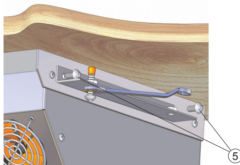
Kiinnitä kiinnitysraudat (3) liedon ruuveilla (5)
